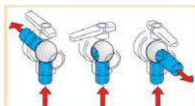
Válvula de Flujo Interrumpido
